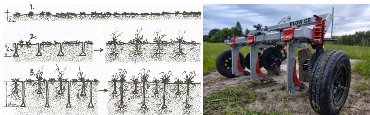
Abb. 6: Keyline Tiefenmeißel.
